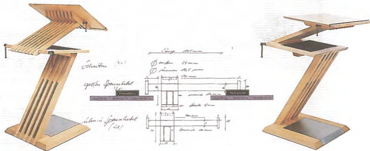
Das Stehpult „Z-LINE“ gibt eine neue Art zu arbeiten vor. Rückenschonend ermöglicht es Lesen und Schreiben. (HASSA TIEDT)
